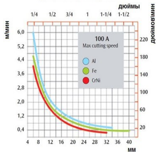
График скорости резания
